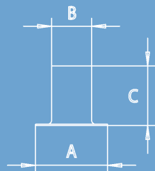
Rivets (détail)
